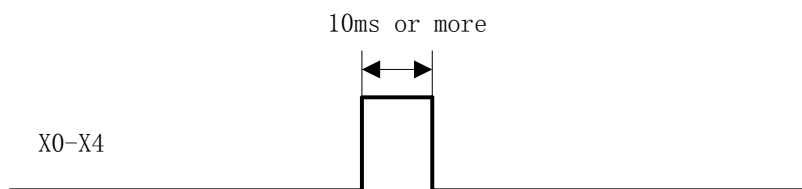
X0-X4 时序图
